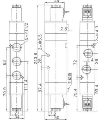
●4V430出线式
