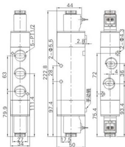
●4V420出线式
