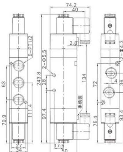
●4V430DIN插座式
